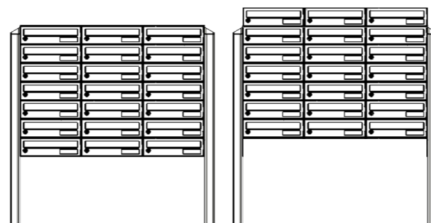
Montagevoorbeeld 21-delig systeem (Terzo-voet & ingebetonneerd)
